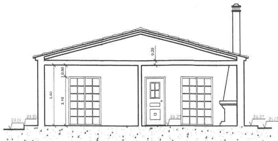
Corte Transversal AA
