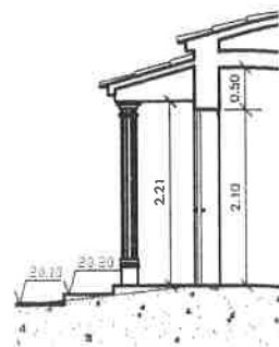
Corte Longitudinal
