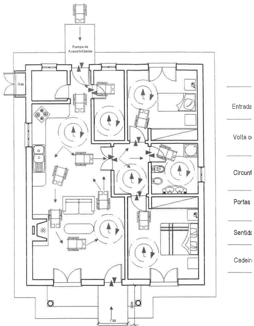
Planta de Apresentação Acessibilidades
