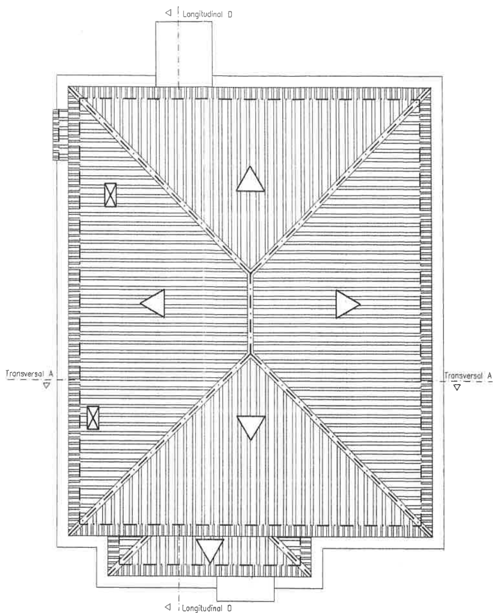
Planta de Cobertura
