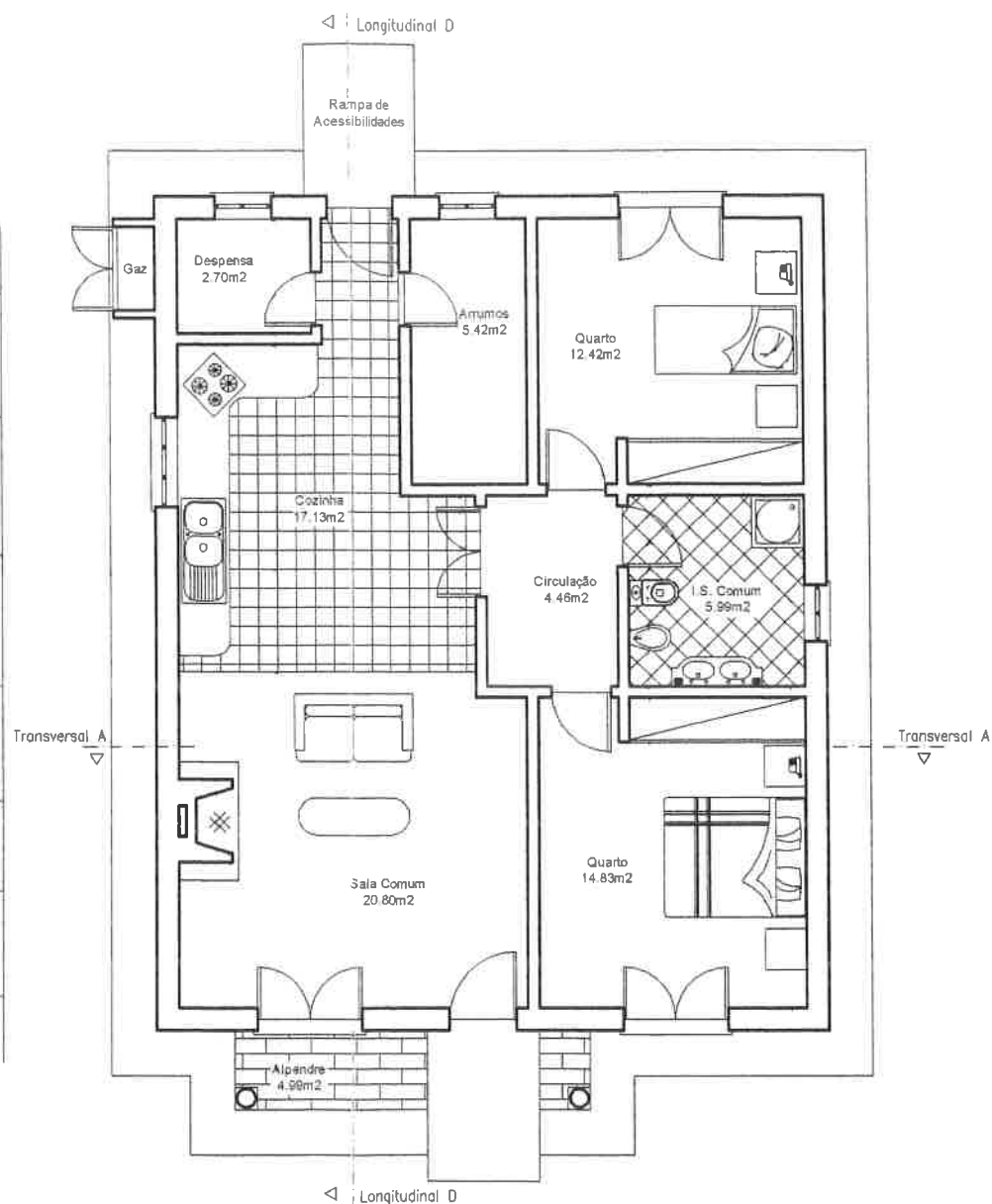
Planta de Apresentação Moradia - 104.88m²
